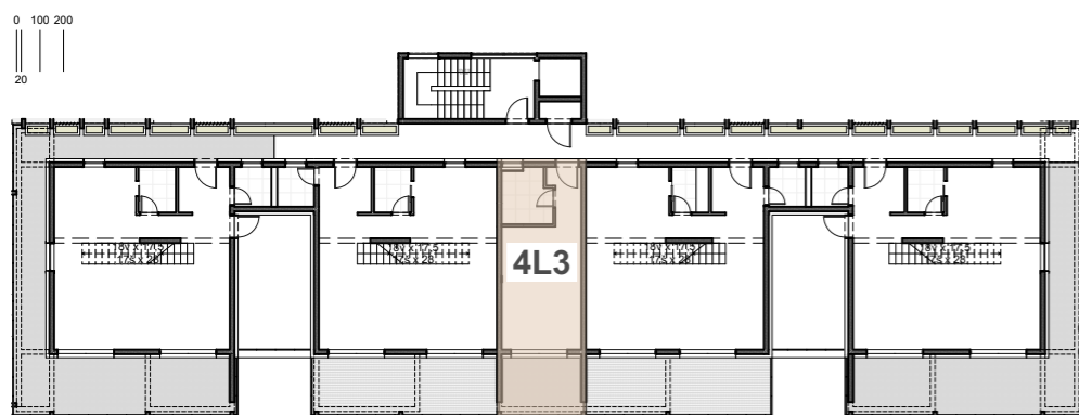
Pozicija stana na etaži 3. kata
