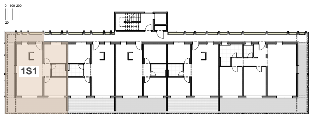
Pozicija stana na etaži 1. kata
